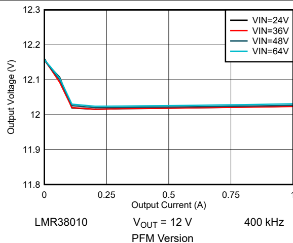
图 9-14. 12-V Load Regulation
