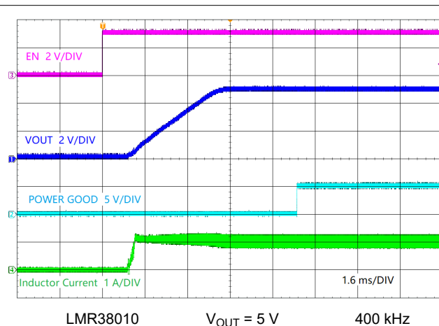
图 9-4. Start-Up by EN
