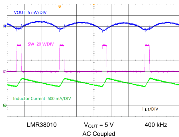
图 9-6. Full Load Switching
