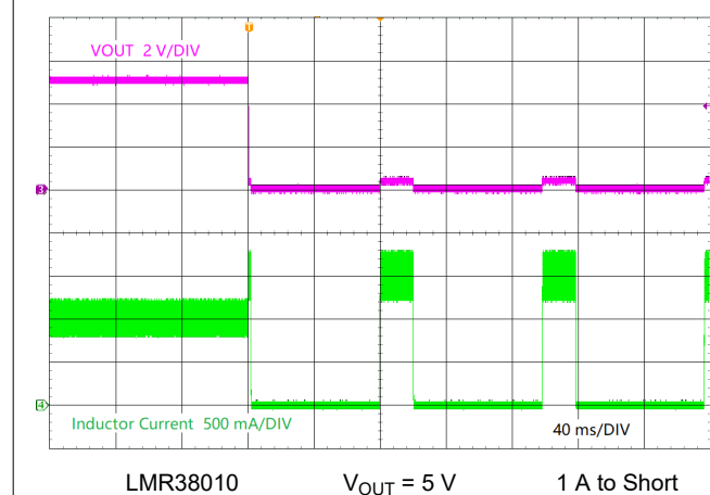
图 9-7. Short Circuit Applied
