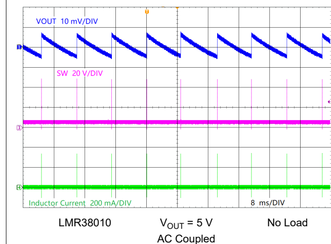
图 9-5. PFM Switching
