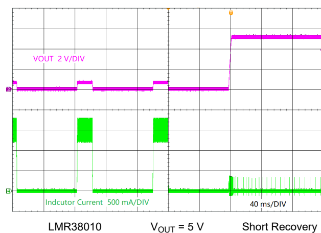
图 9-8. Short-Circuit Recovery
