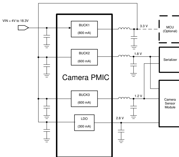
TPS650320-Q1 应用电路
