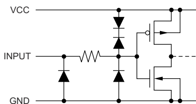
图 7-1. SIN, SCLK, LAT, GSCLK
