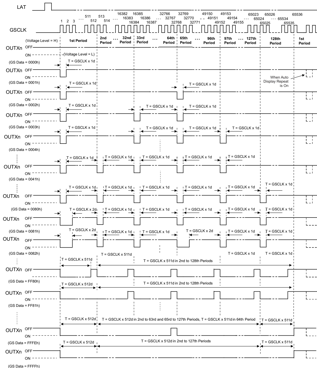
图 8-8. ES PWM Operation
