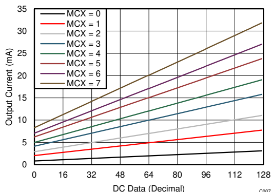
图 6-7. Dot Correction (DC) Linearity
