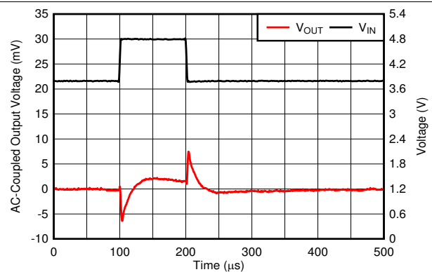
图 6-33. Line Transient
