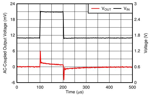
图 6-31. Line Transient
