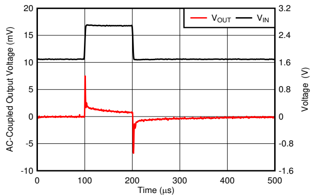
图 6-31. Line Transient
