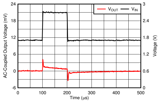
图 6-26. Line Transient
