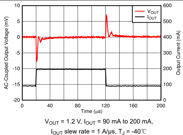
图 6-54. Load Transient
