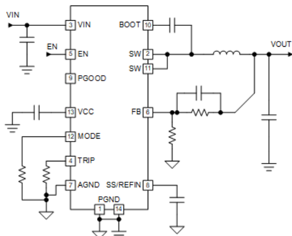
简化原理图
