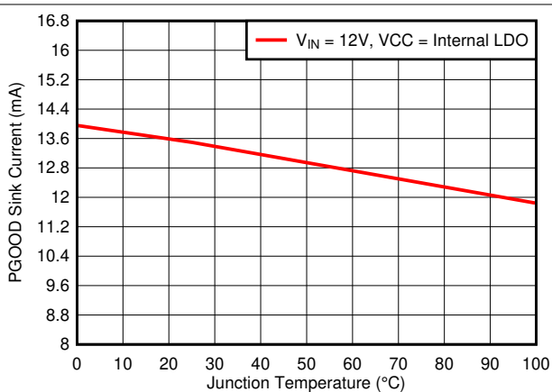
图 5-10. PGOOD 灌电流
