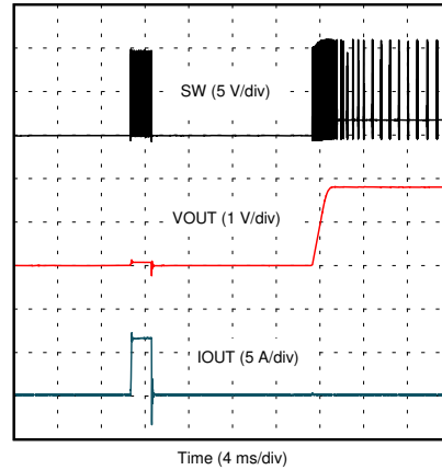
图 7-32. 过流退出断续模式
