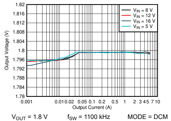
图 7-11. 输出电压与输出电流间的关系 - DCM
