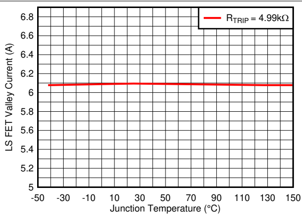
图 5-3. 过流限值
