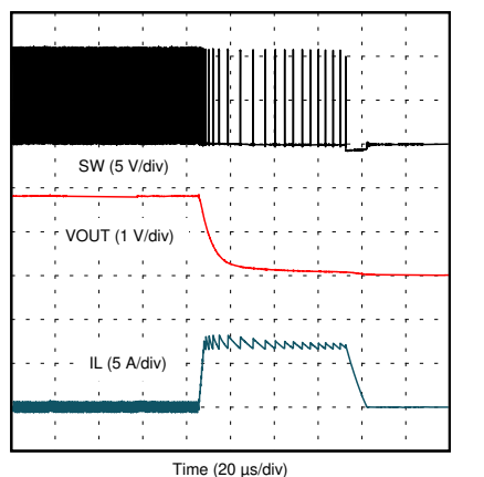
图 7-28. 过流响应
