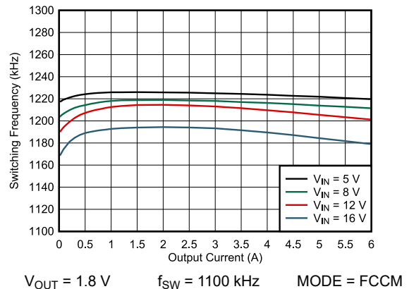
图 7-13. 开关频率与输出电流间的关系 - 1100kHz
