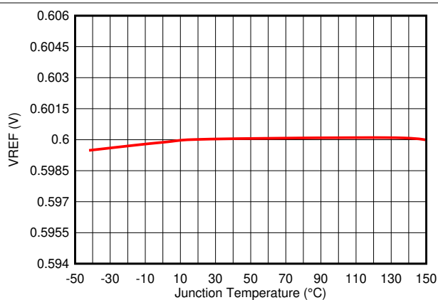
图 5-6. Vref
