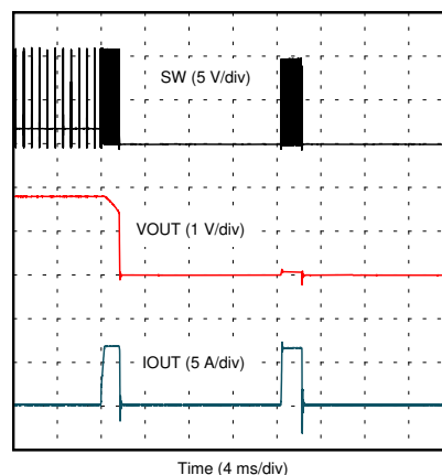
图 7-29. 过流响应
