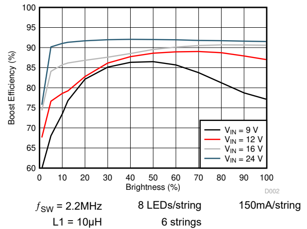
图 5-3. Boost Efficiency
