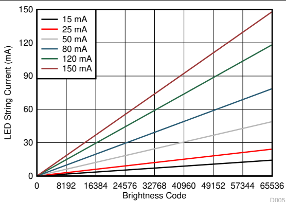
图 5-6. Current Linearity
