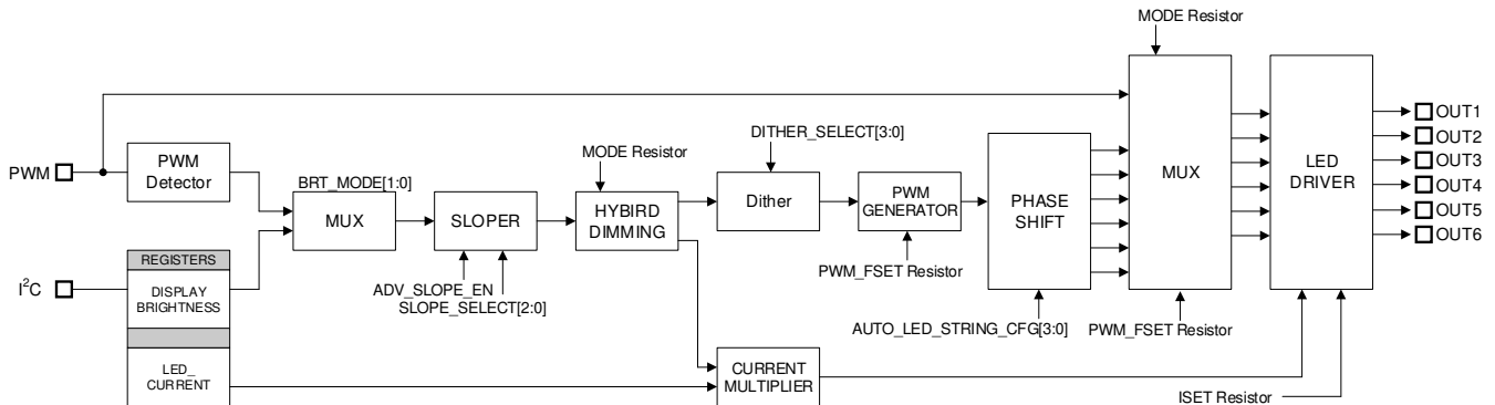
图 6-9. LP8866-Q1 Brightness Path Diagram
