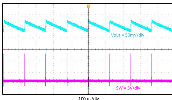
图 8-5. 输出电压纹波, 10mA
