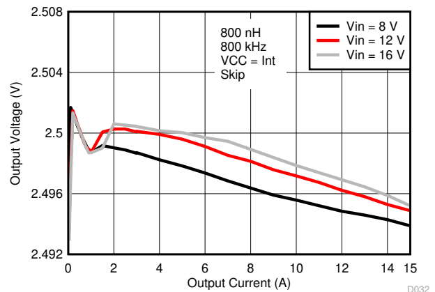
图 8-7. 输出电压与输出电流间的关系
