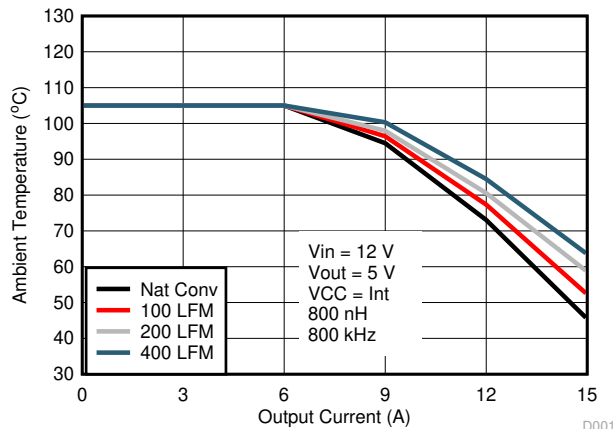
图 6-5. 安全工作区， V_{OUT} = 5\text{V}
