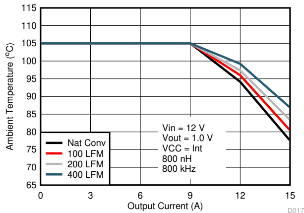
图 6-3. 安全工作区， V_{OUT} = 1.0\text{V}
