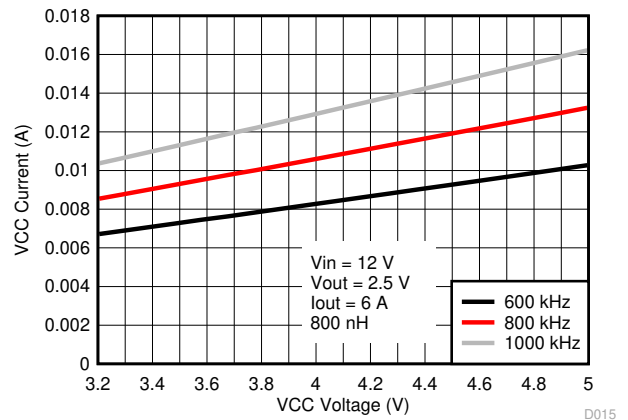
图 8-13. ICC 电流与外部 VCC 电压间的关系
