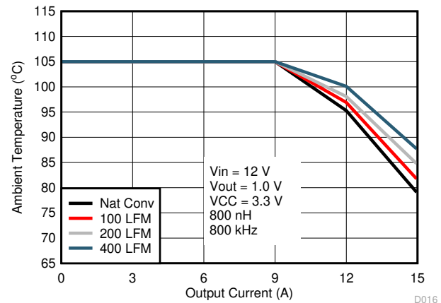
图 6-4. 安全工作区， V_{OUT} = 1.0\text{V}
