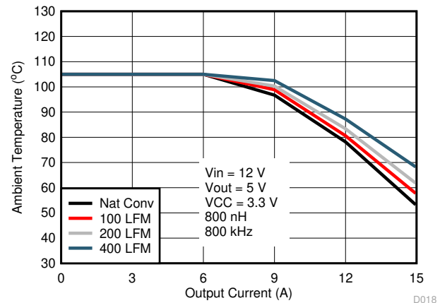
图 6-6. 安全工作区， V_{OUT} = 5\text{V}
