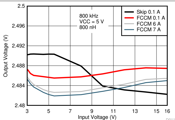
图 8-12. 输出电压与输入电压间的关系, VCC = 5.0V 外部偏置
