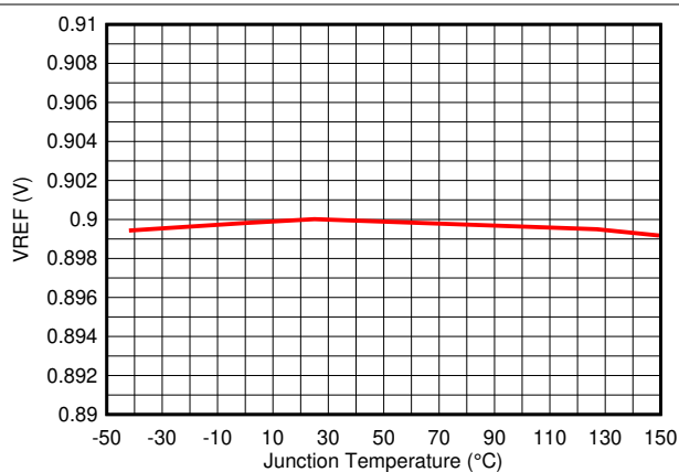
图 5-6. Vref
