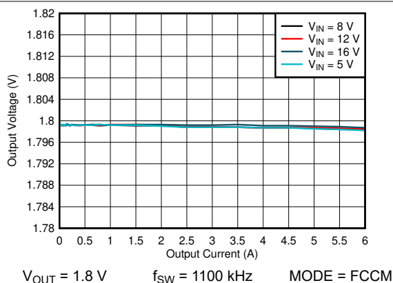
图 7-10. 输出电压与输出电流间的关系 - FCCM
