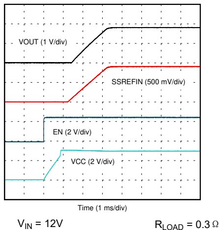
图 7-16. EN 启动
