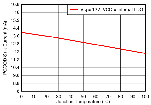
图 5-10. PGOOD 灌电流
