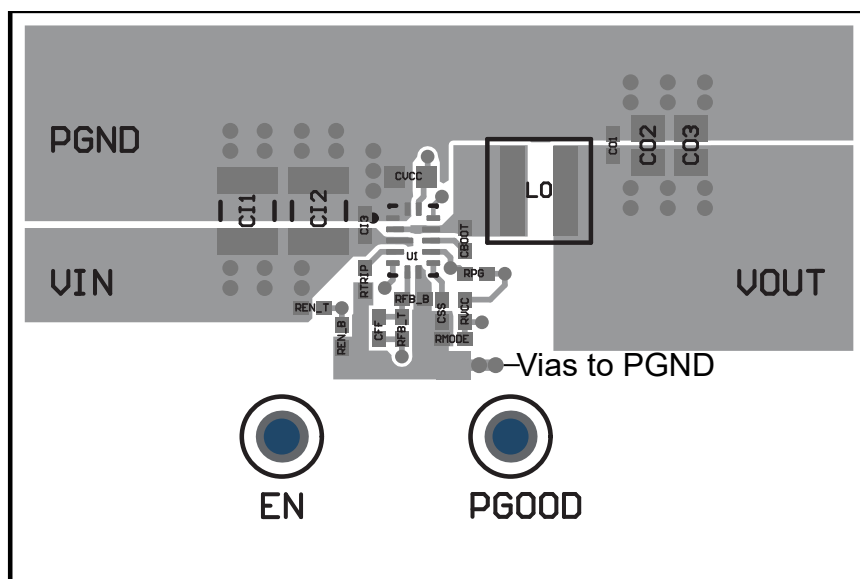
图 7-31. 顶层布局
