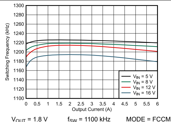
图 7-13. 开关频率与输出电流间的关系 - 1100kHz
