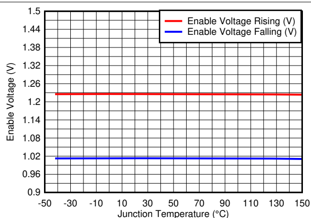
图 5-5. 使能电压
