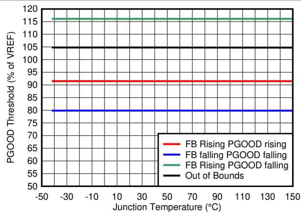
图 5-9. PGOOD 阈值
