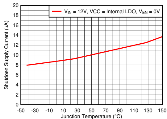
图 5-14. 关断电源电流
