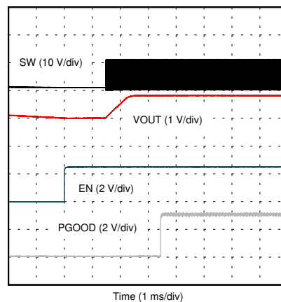
图 7-27. 以预偏置进行 EN 启动
