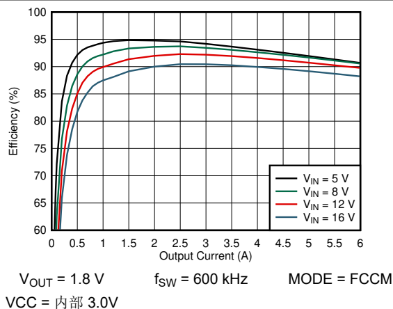
图 7-8. 效率 - 600kHz, FCCM
