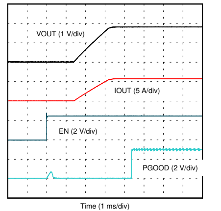
图 7-15. EN 启动
