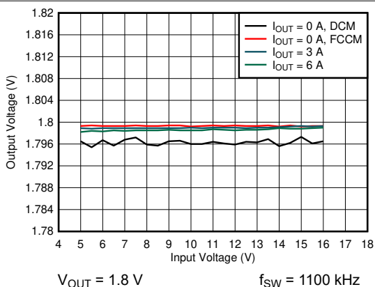
图 7-12. 输出电压与输入电压间的关系
