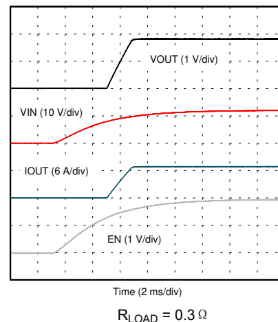
图 7-19. V_{IN} 启动
