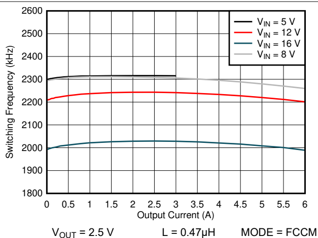
图 5-17. 2200kHz 开关频率与负载电流间的关系
