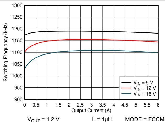
图 5-16. 1100kHz 开关频率与负载电流间的关系
