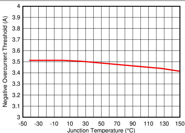
图 5-4. 负过流限制
