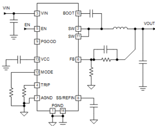
简化原理图
