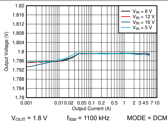
图 7-11. 输出电压与输出电流间的关系 - DCM
