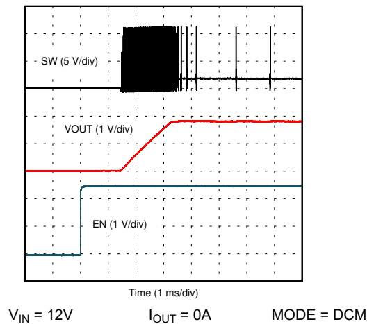
图 7-17. EN 启动 - DCM
