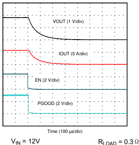
图 7-18. EN 关断
