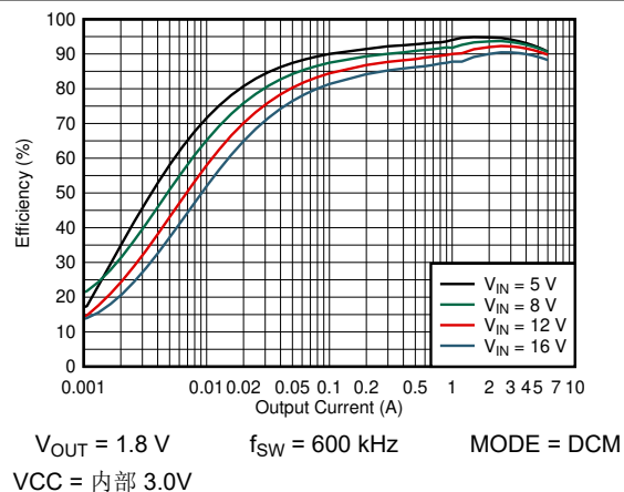
图 7-9. 效率 - 600kHz, DCM
