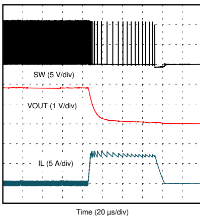
图 7-30. 短路响应
