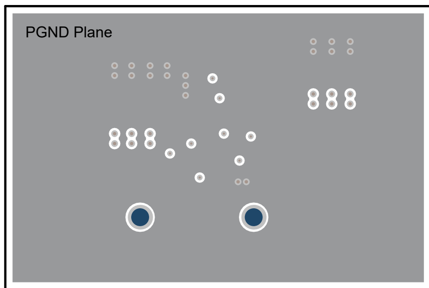
图 7-32. 信号层 1 布局
