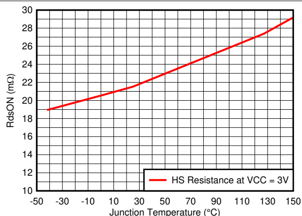
图 5-1. 高侧 FET RdsON
