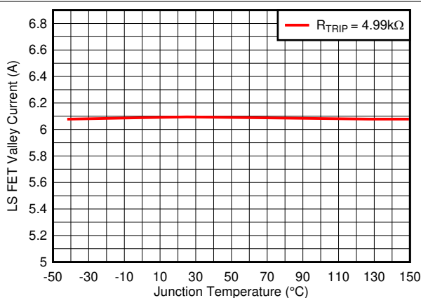
图 5-3. 过流限值
