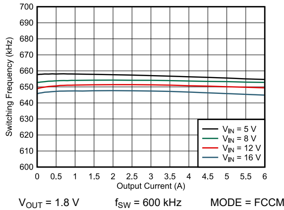
图 7-14. 开关频率与输出电流间的关系 - 600kHz
