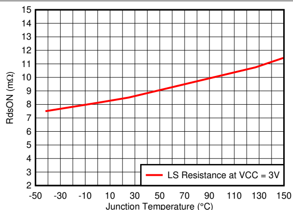
图 5-2. 低侧 FET RdsON
