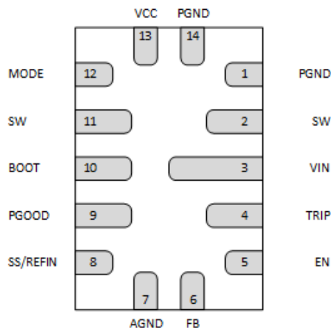
图 4-2. 14 引脚 VQFN-HR、RPG 封装 ( 底视图 )
