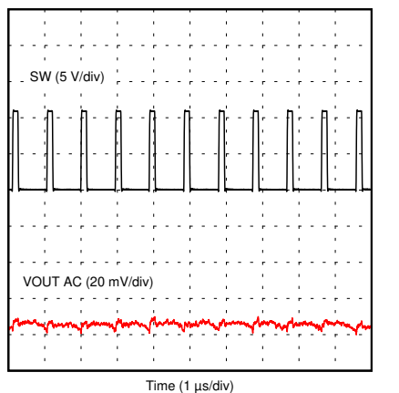
图 7-26. 输出电压纹波
