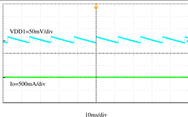
图 8-11. VDD1 Output Voltage Ripple, I_{OUT} = 0\text{ A}
