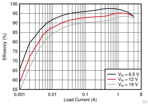
图 18. Efficiency
