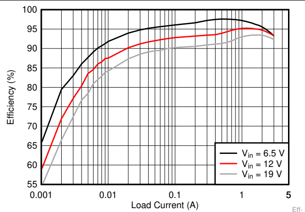
图 11. V_{OUT}=1.05\text{ V} Efficiency, L=1.5\text{ }\mu\text{H}
