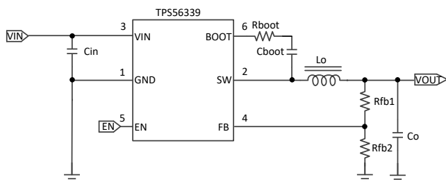
简化原理图
