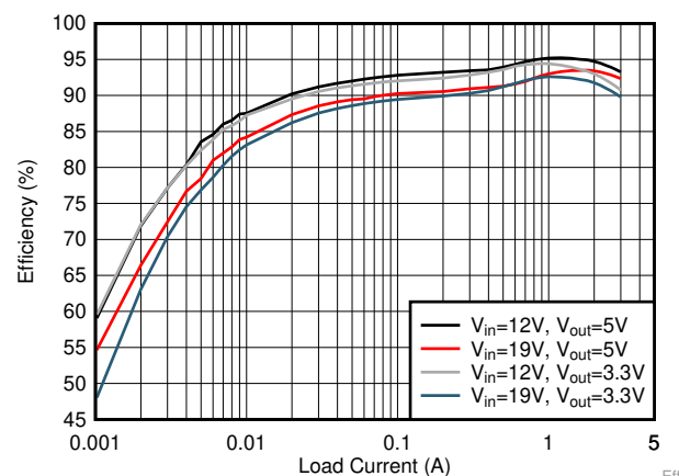
TPS56339 效率
