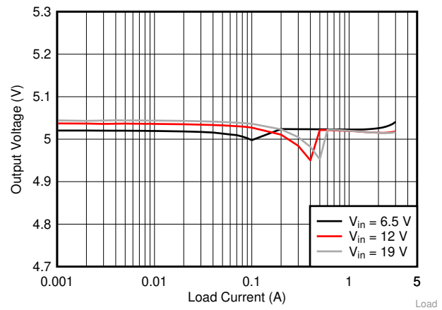
图 19. Load Regulation
