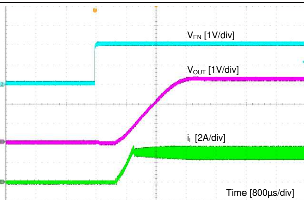
图 16. PSM Mode
