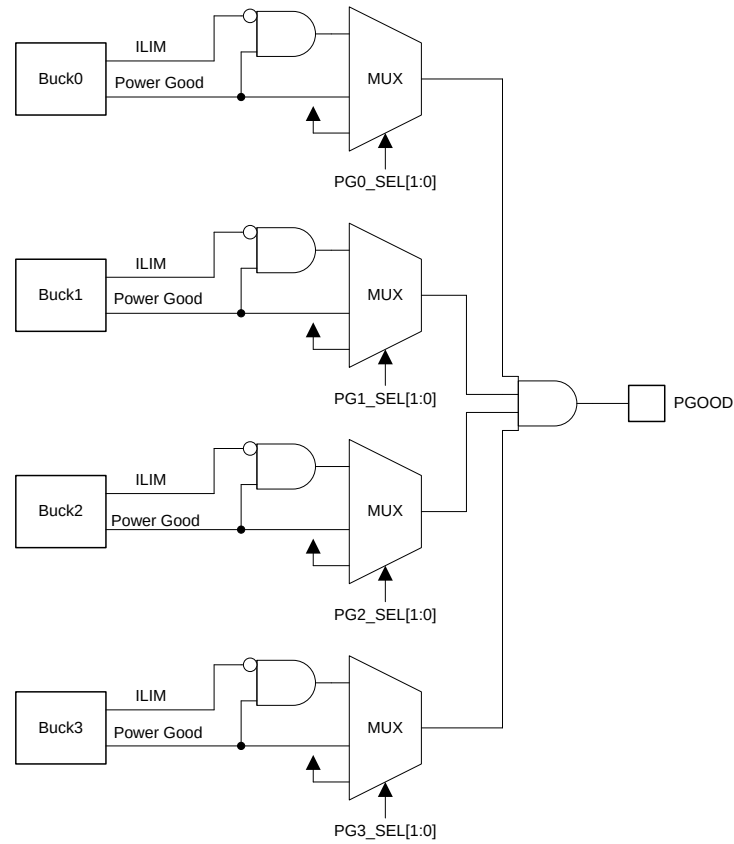
图 18. PGOOD Block Diagram
