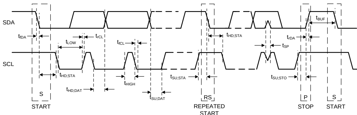
图 24. I²C-Compatible Timing
