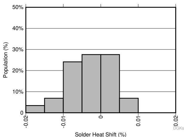
图 9-3. 焊接热漂移分布， V_{REF} (%) - DGK 封装
