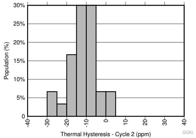
图 9-9. 热迟滞分布 ( V_{REF} ) - DGK 封装 (周期 2)
