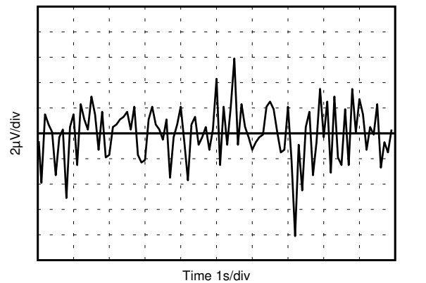
图 8-24. 0.1Hz 至 10Hz 噪声 ( V_{REF} )
