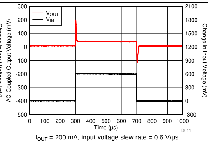
图 18. V_{IN} Transient
