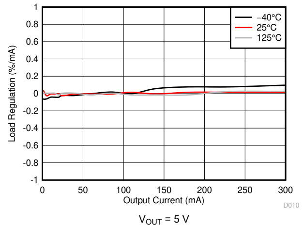
图 6-10. Load Regulation
