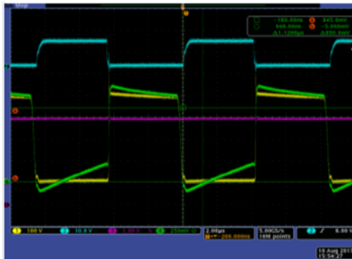
CH1 = V_{DS} CH2 = V_{DR} CH3 = V_{CO}
