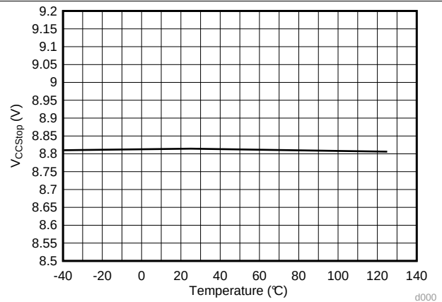
图 2. VCCStop 阈值与温度间的关系
