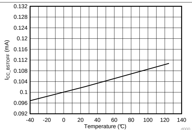
图 4. VCC 启动电流与温度间的关系
