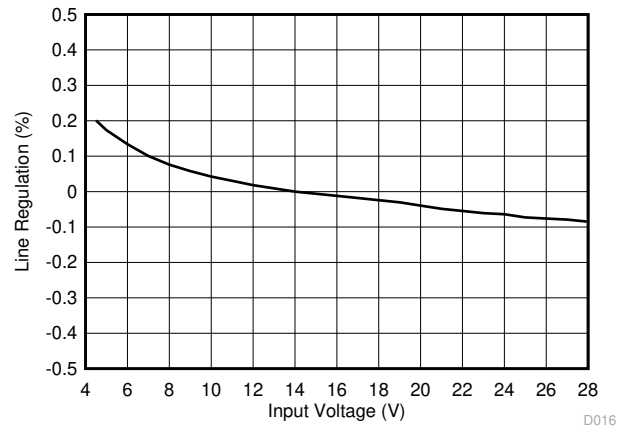
图 8-3. 线路调节
