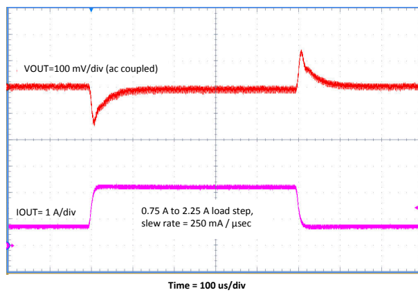
图 8-11. 瞬态响应
