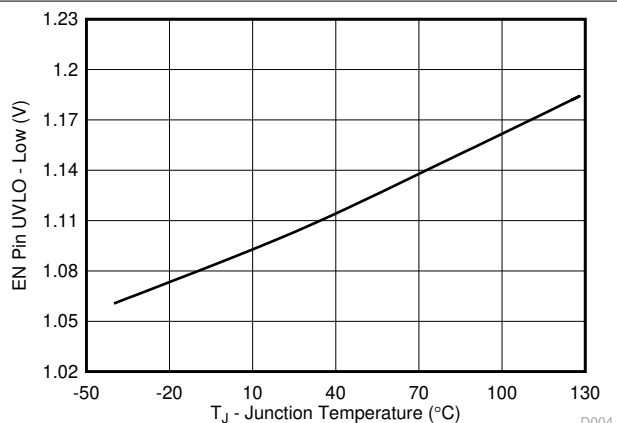
图 6-3. EN Pin UVLO Low Voltage vs Junction Temperature
