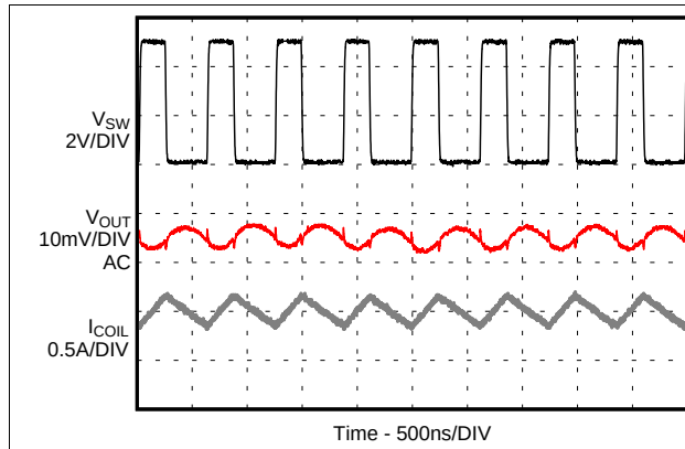
图 14. PWM Operation
