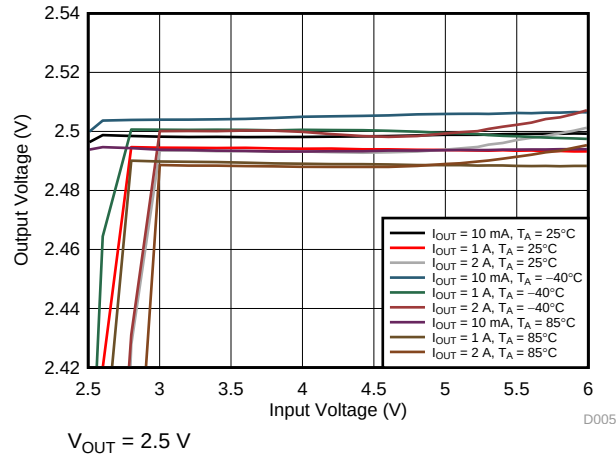
图 5. Output Voltage vs Input Voltage
