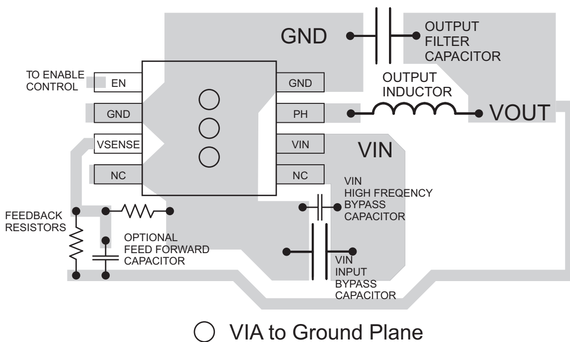
图 19. Layout Schematic
