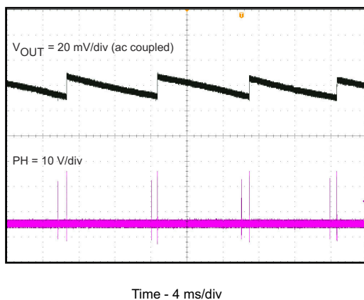
图 8-6. 输出电压纹波
