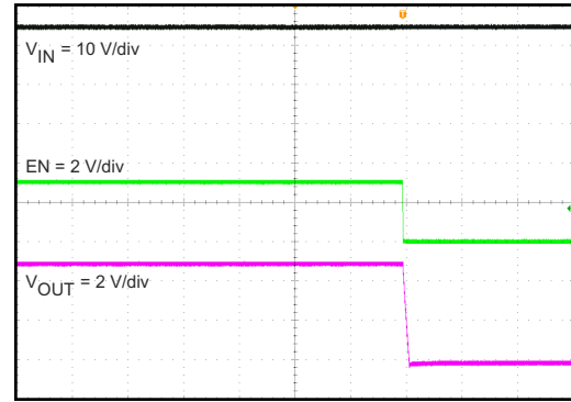
Time - 2 ms/div 图 8-15. 相对于 EN 的关断
