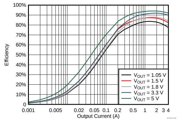
TPS564208 效率
