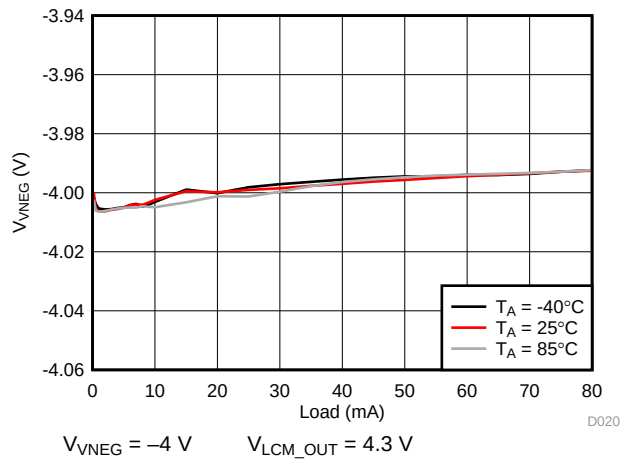
图 23. V_{VNEG} Load Regulation
