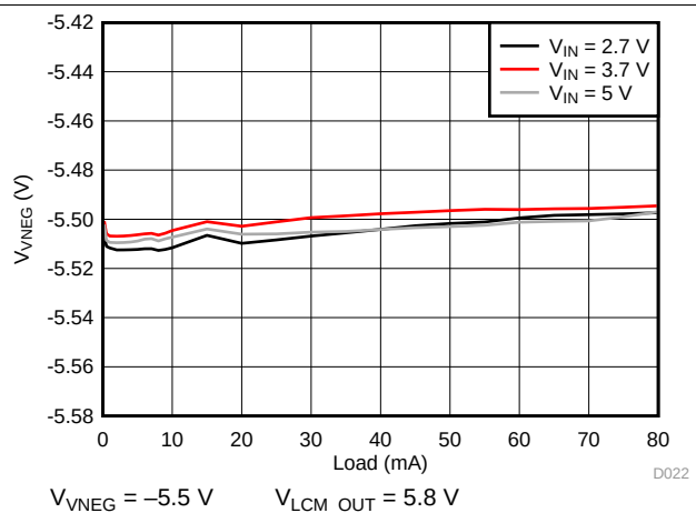
图 25. V_{VNEG} Load Regulation
