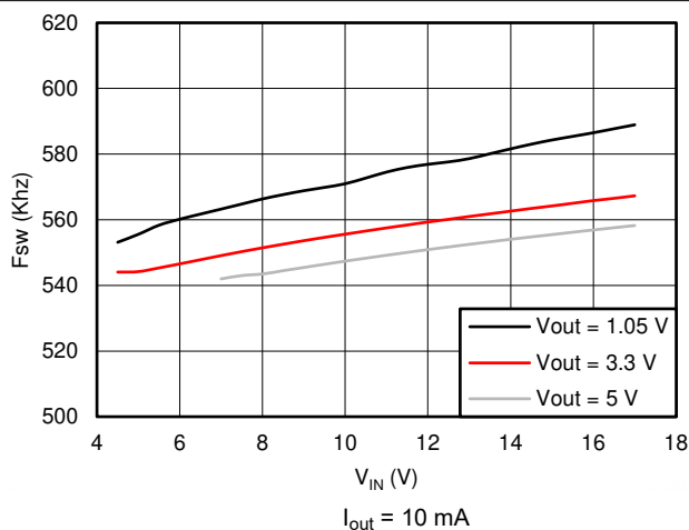
图 5-7. TPS562208 Switching Frequency vs Input Voltage
