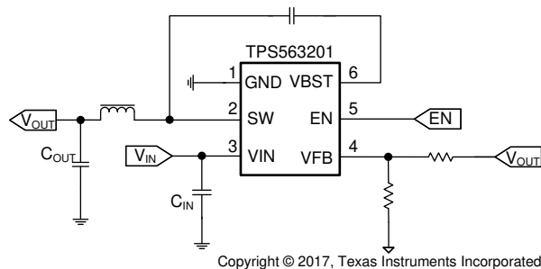
简化原理图
