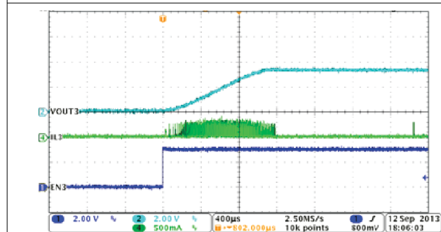
图 8-7. PSM Mode Buck3, Soft-Start With No Load
