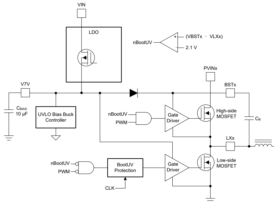
图 7-4. V7V 线性 Dropout 调节器和 Bootstrap 电压图
