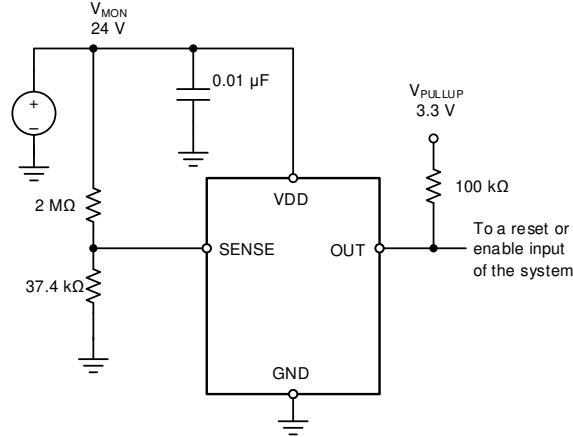
图 7-3. 24-V, 10% Comparator
