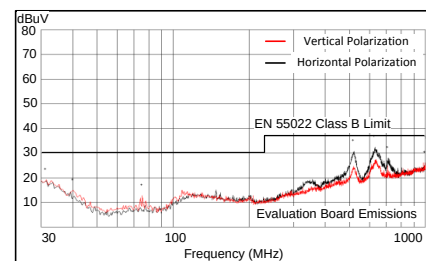
辐射发射图
