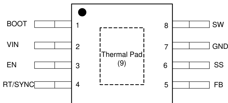
图 5-1. DDA 封装 8 引脚 SOIC 俯视图
