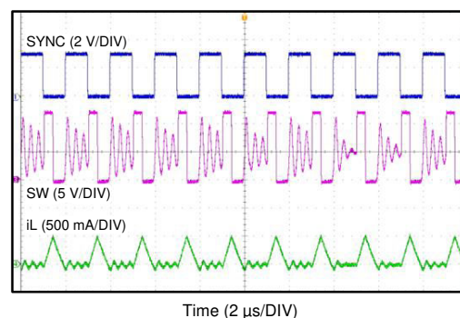
图 7-7. 在 DCM 下同步
