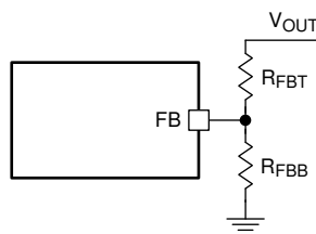
图 7-2. 输出电压设置
