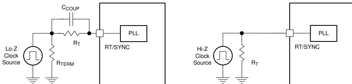
图 7-5. 与外部时钟同步
