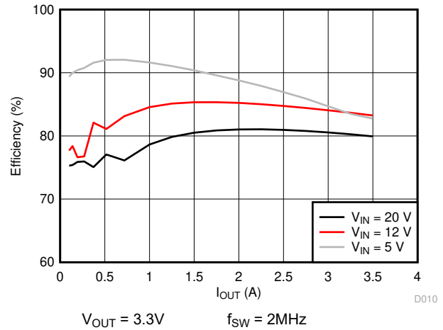
图 6-4. 效率与负载电流间的关系
