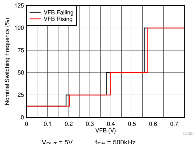
图 6-6. 频率与 V_{FB} 间的关系
