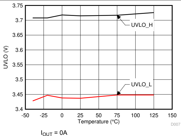
图 6-12. UVLO 阈值
