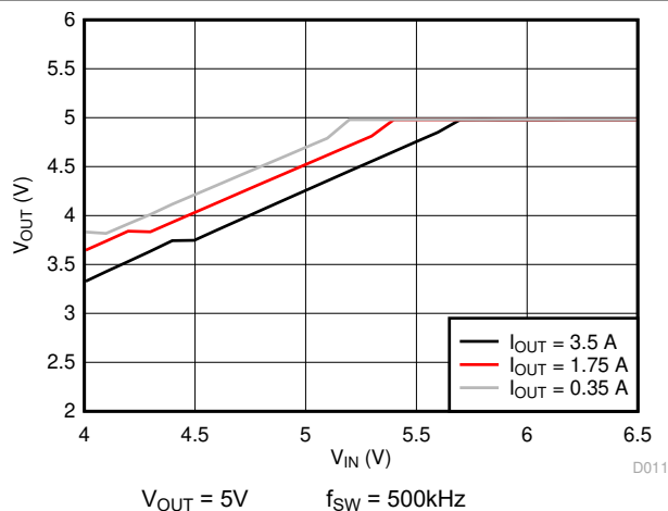
图 6-7. 压降曲线
