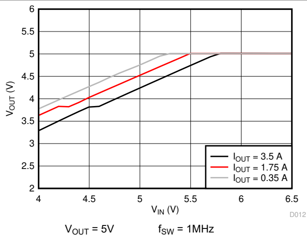
图 6-8. 压降曲线
