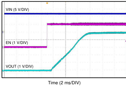
图 8-2. 由 EN 启动
