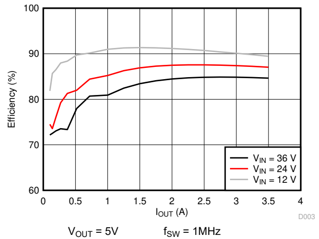
图 6-2. 效率与负载电流间的关系
