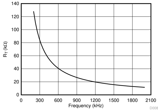
图 7-4. R_T 与频率曲线间的关系
