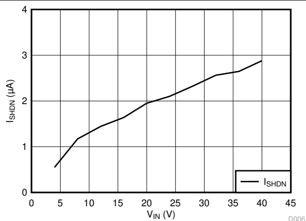
图 6-11. 关断电流
