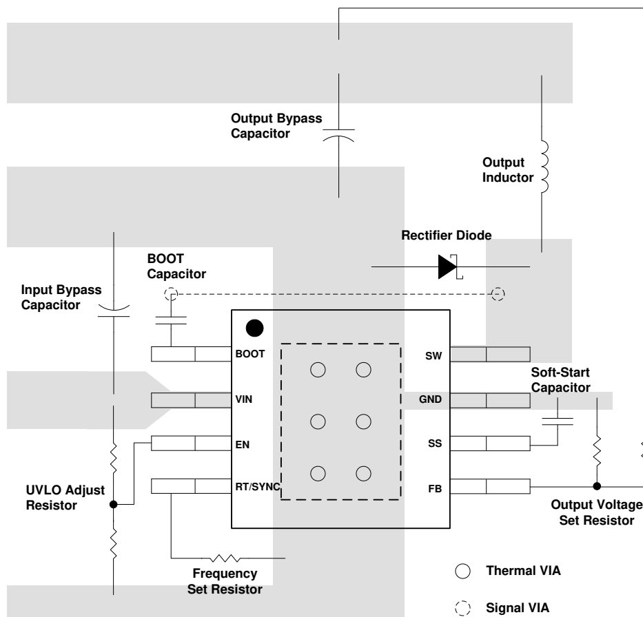
图 8-10. 布局示例
