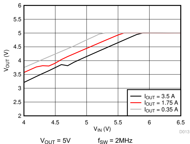
图 6-9. 压降曲线
