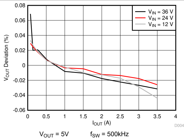
图 6-5. 负载调节
