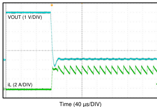
图 8-8. 输出短路
