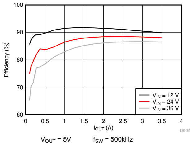
图 6-1. 效率与负载电流间的关系
