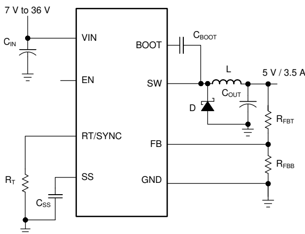
图 8-1. 应用电路，5V 输出
