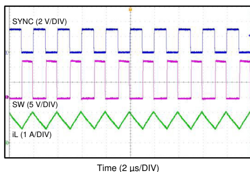
图 7-6. 在 CCM 下同步
