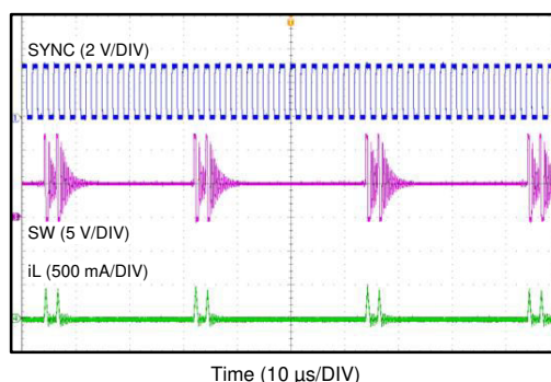
图 7-8. 在 PSM 下同步
