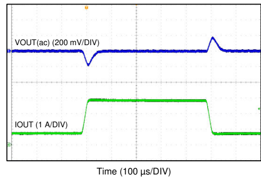
图 8-5. DCM 模式
