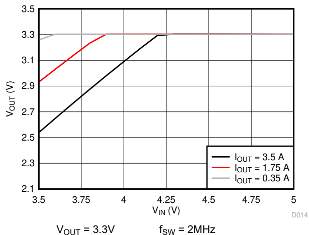
图 6-10. 压降曲线
