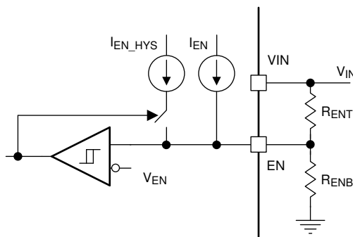
图 7-3. 由使能分压器实施的系统 UVLO
