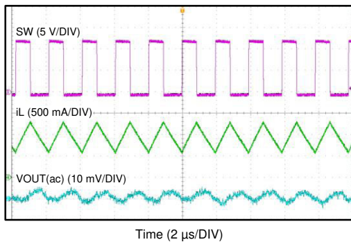
图 8-6. CCM 模式
