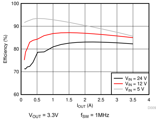
图 6-3. 效率与负载电流间的关系
