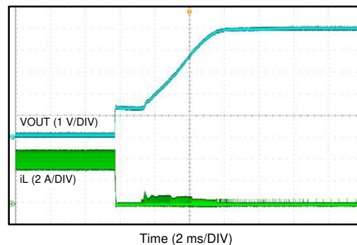
图 8-9. 输出短路恢复
