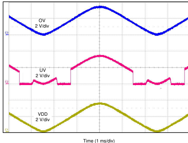
图 7-7. TPS3702CX33-Q1 Window Voltage Detector Function
