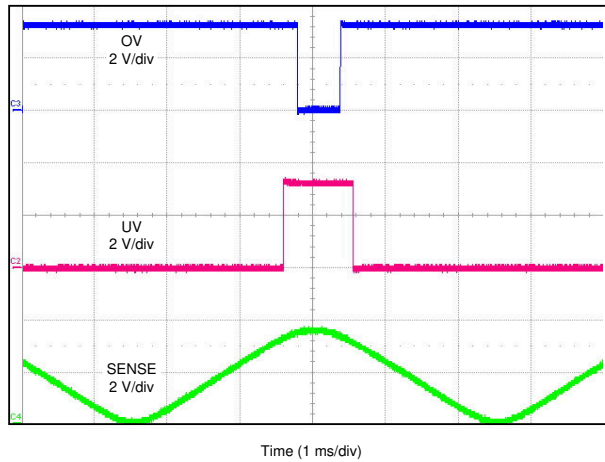
图 7-7. TPS3702CX33-Q1 Window Voltage Detector Function
