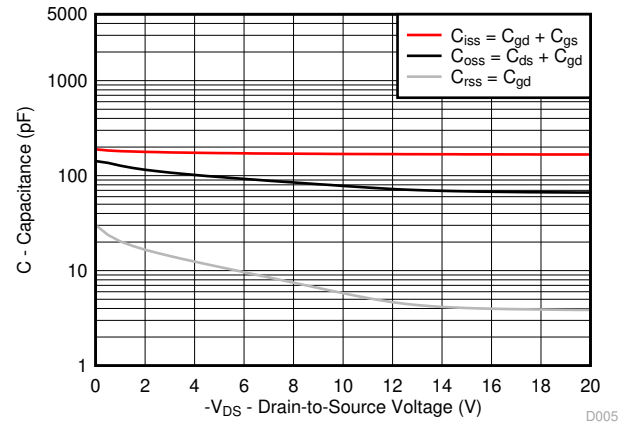
图 5-5. Capacitance
