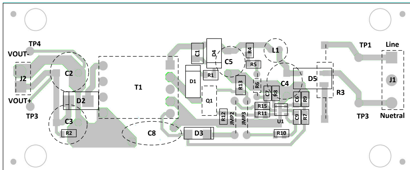
图 10-2. Layout Example
