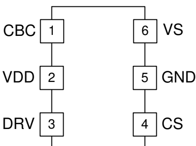
图 5-1. UCC28700-Q1 SOT23-6 (DBV) Top View
