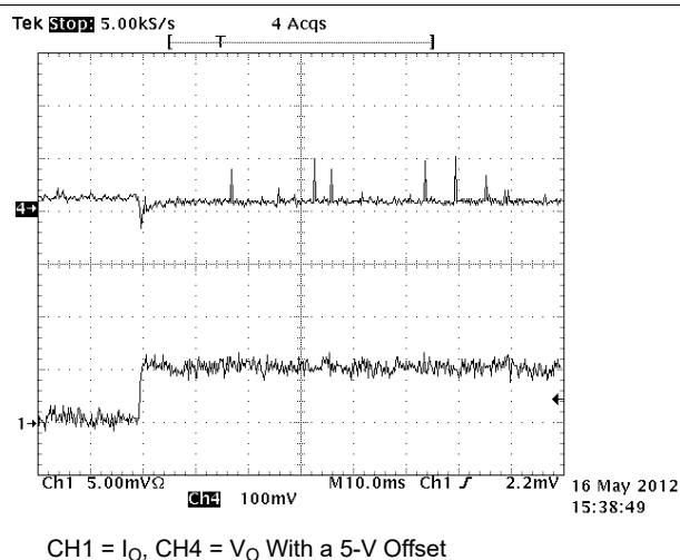
图 8-6. Load Transients: (0.1-A to 0.6-A Load Step)
