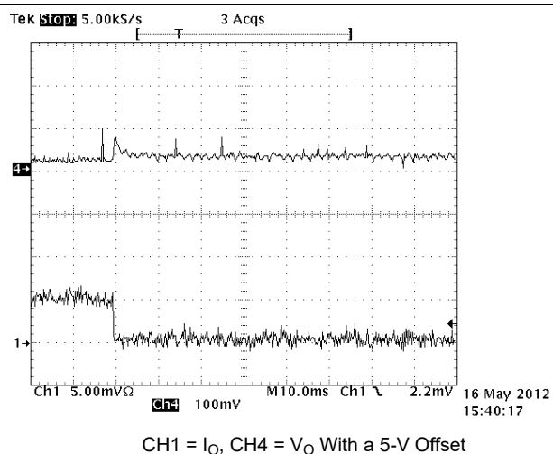
图 8-7. Load Transients: (0.6-A to 0.1-A Load Step)
