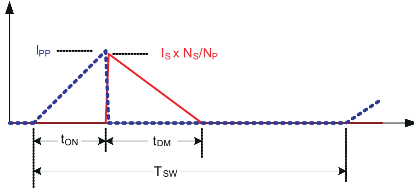
图 7-5. Transformer Currents
