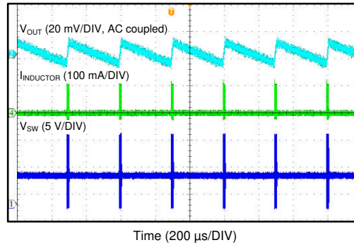
图 8-10. Eco-mode Operation
