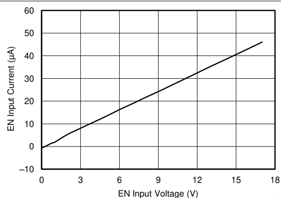
图 6-13. En Current vs En Voltage
