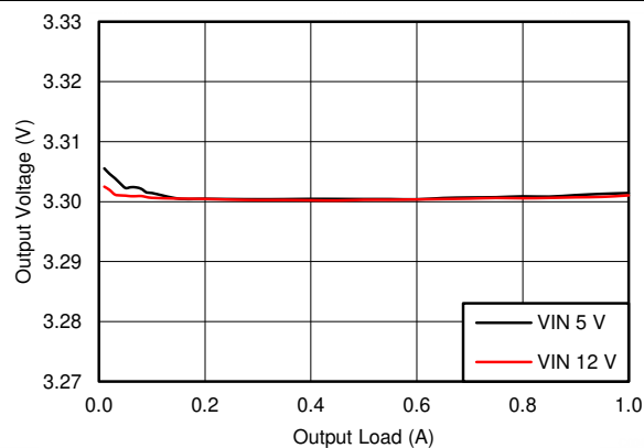
图 7-5. BUCK3, Load Regulation
