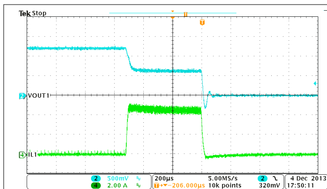
图 9-20. Buck1, OCP
