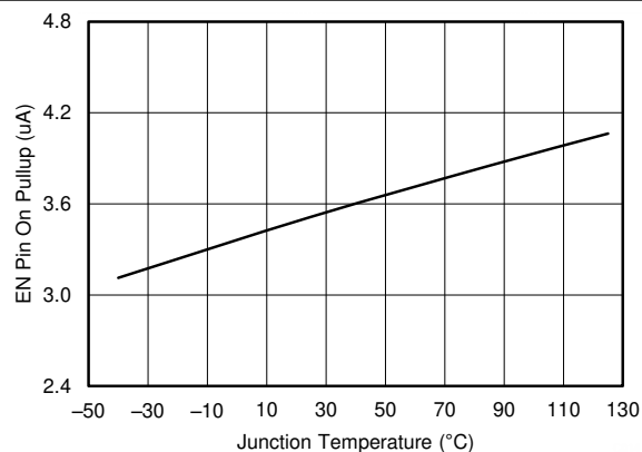
图 7-16. EN Pin Pullup Current vs Temperature, EN = 1 V
