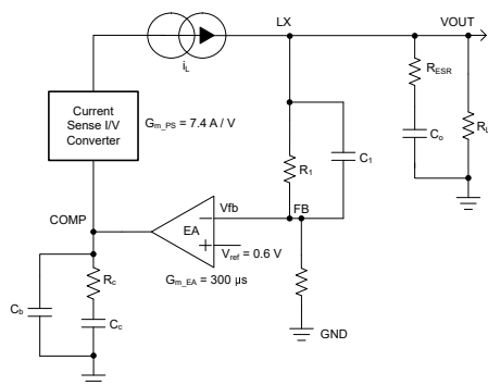
图 9-1. DC/DC Loop Compensation
