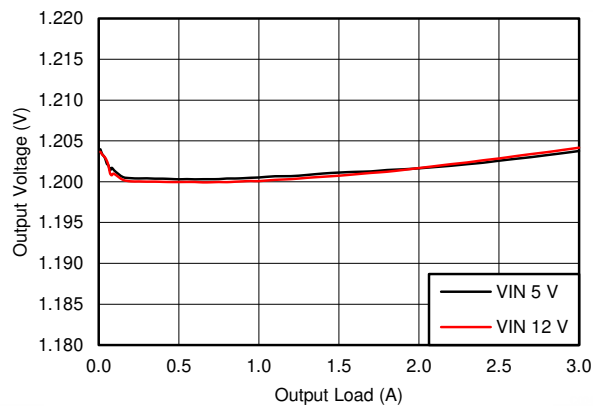
图 7-3. BUCK1, Load Regulation
