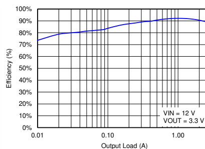
效率与输出负载之间的关系
