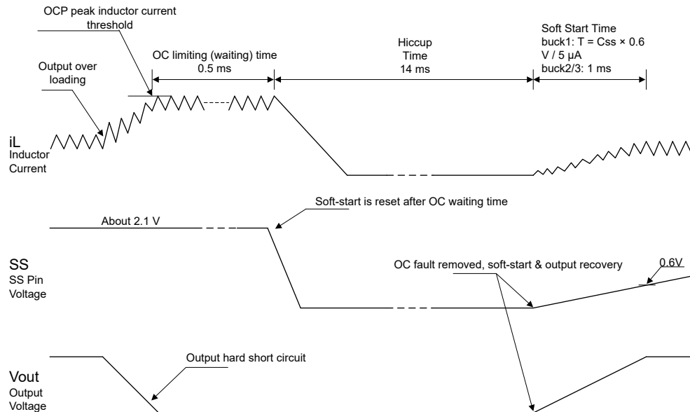
图 8-7. OCP
