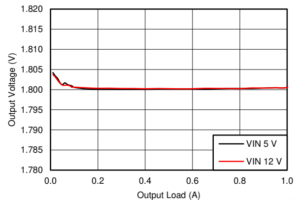
图 7-4. BUCK2, Load Regulation
