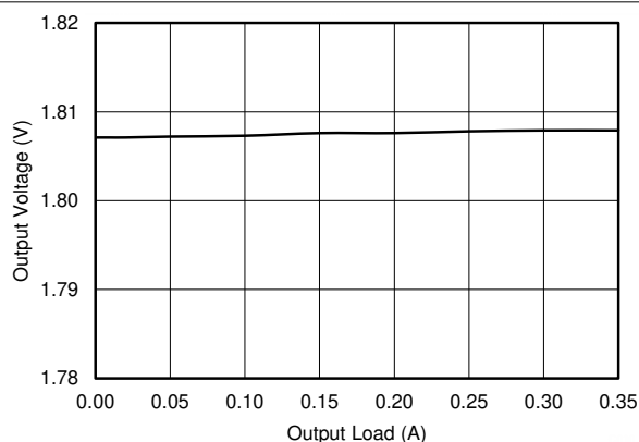
图 7-9. LDO1, Load Regulation
