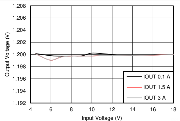
图 7-6. BUCK1, Line Regulation
