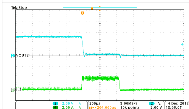
图 9-24. Buck3, OCP
