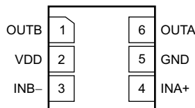
图 5-2. DSE Package WSON-6 Top View
