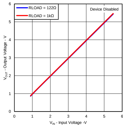
图 9. Output Voltage vs Input Voltage
