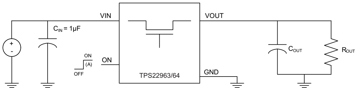
图 36. Test Circuit
