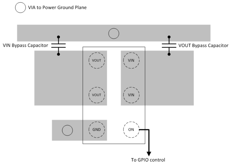
图 43. Layout Example
