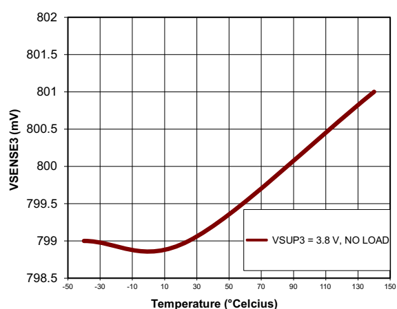
图 7-10. Buck3 = 1.2-V VSENSE3 vs Temperature EXTSUP Pin Open
