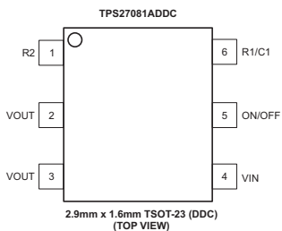
图 1. TPS27081A 封装
