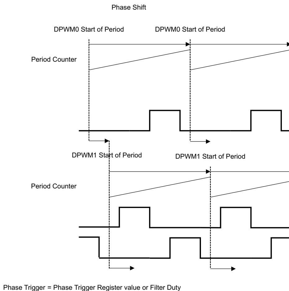
图 9-18. Phase Shift
