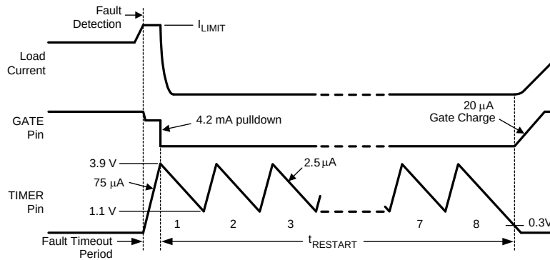
图 24. Restart Sequence
