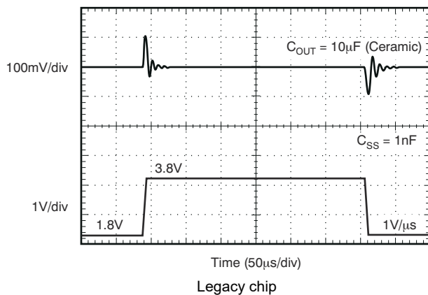
图 5-33. V_{IN} Line Transient
