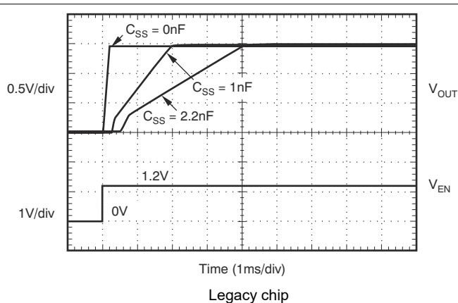
图 5-37. Turn-On Response
