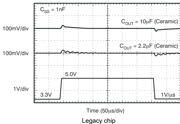
图 5-31. V_{BIAS} Line Transient
