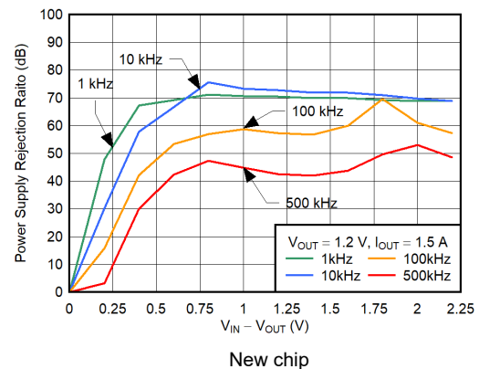
图 5-18. V_{IN} PSRR vs (V_{IN} - V_{OUT})
