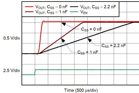
图 7-3. Turn-On Response
