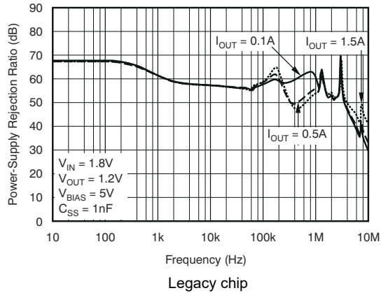
图 5-13. V_{BIAS} PSRR vs Frequency
