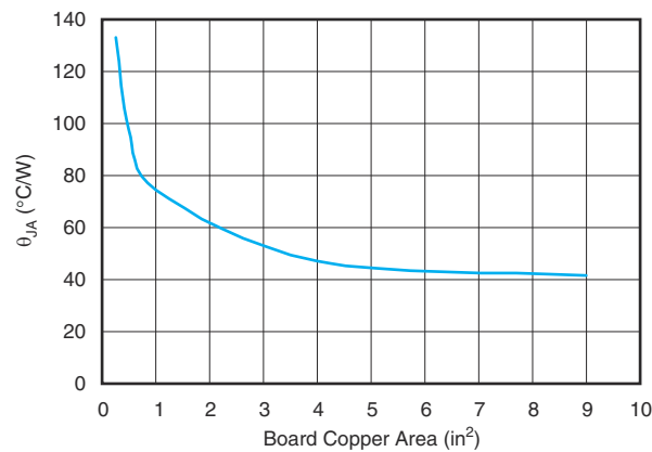
图 7-4. R_{\theta JA} vs Board Size
