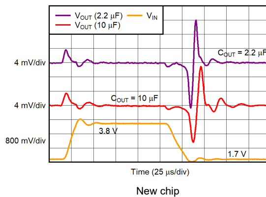
图 5-34. V_{IN} Line Transient
