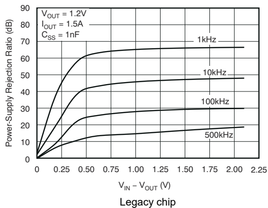
图 5-17. V_{IN} PSRR vs (V_{IN} - V_{OUT})
