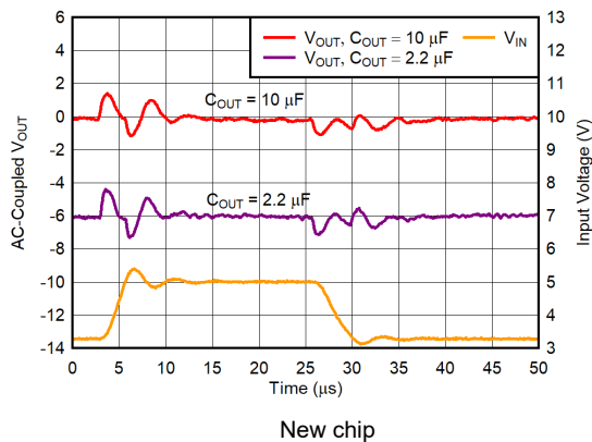
图 5-32. V_{BIAS} Line Transient
