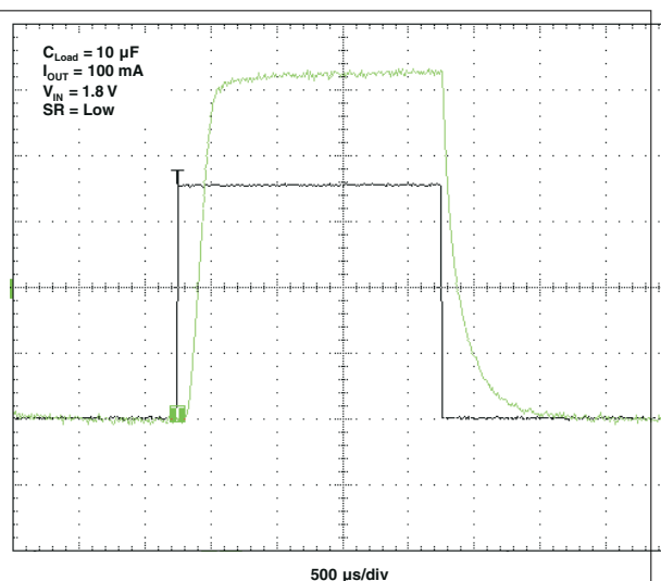
图 5-21. t_{ON} Response
