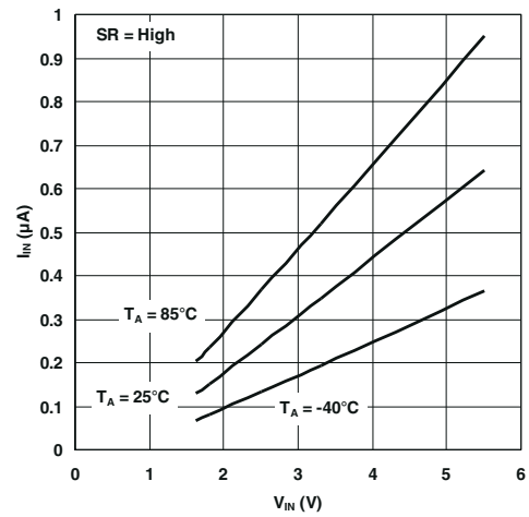
图 5-4. Quiescent Current vs Input Voltage
