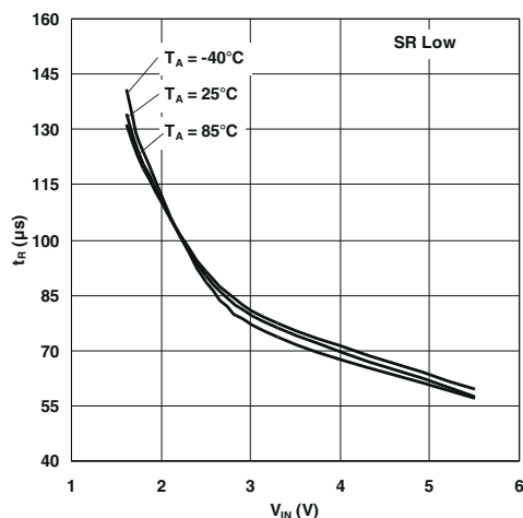
图 5-7. Rise Time vs Input Voltage
