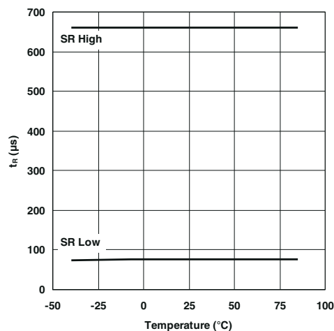
图 5-9. Rise Time vs Temperature
