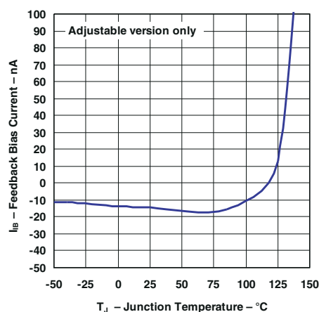
图 6-10. FEEDBACK Current
