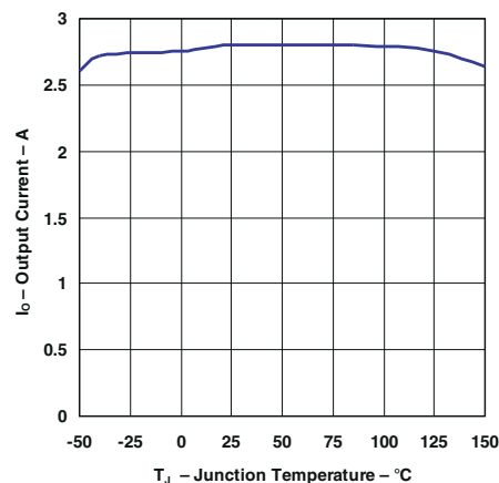
图 6-4. Current Limit
