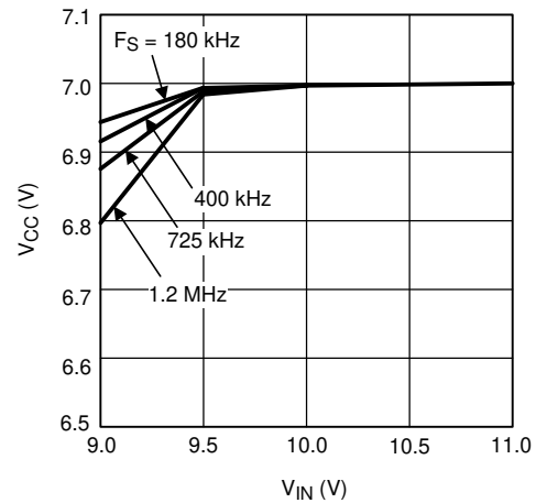
图 6-2. V_{CC} vs V_{IN} and F_S
