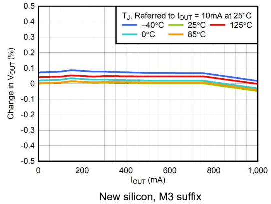
图 5-2. Load Regulation
