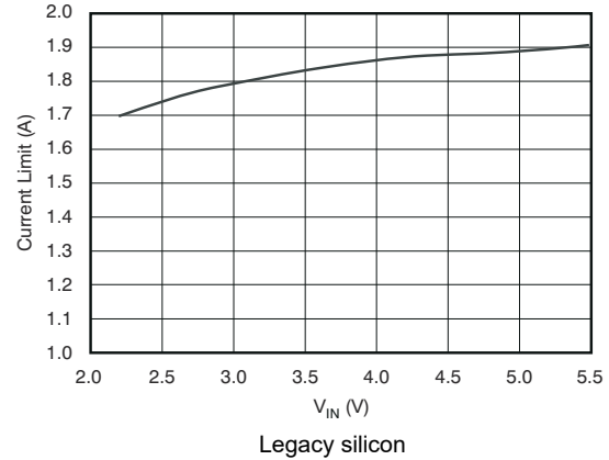
图 5-18. Current Limit vs V_{IN}
