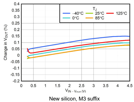
图 5-4. Line Regulation
