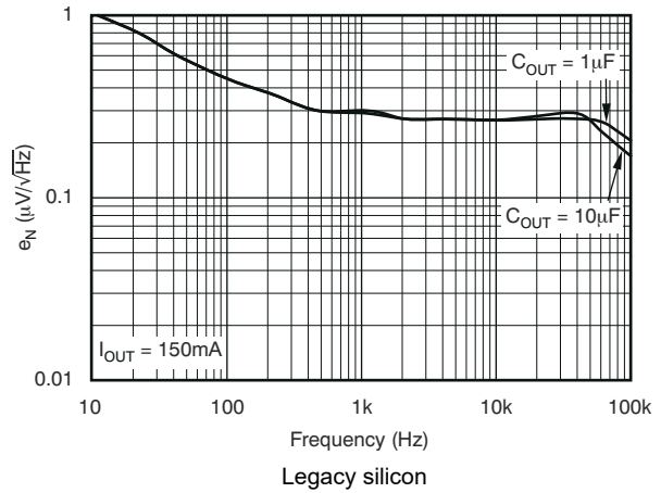
图 7-4. Noise Spectral Density
