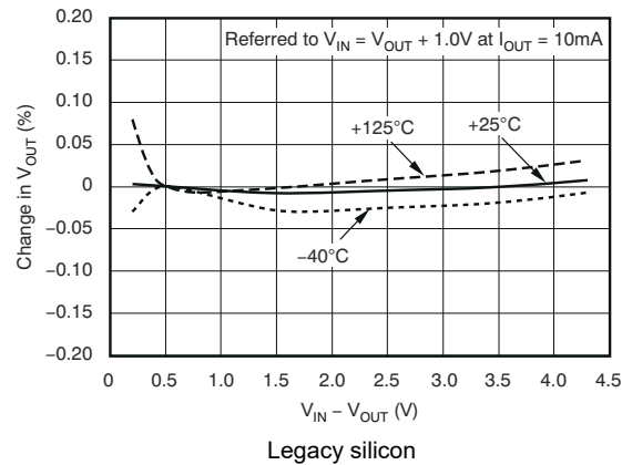
图 5-3. Line Regulation
