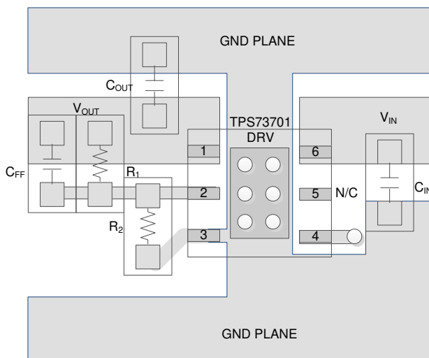
图 7-9. Layout Example
