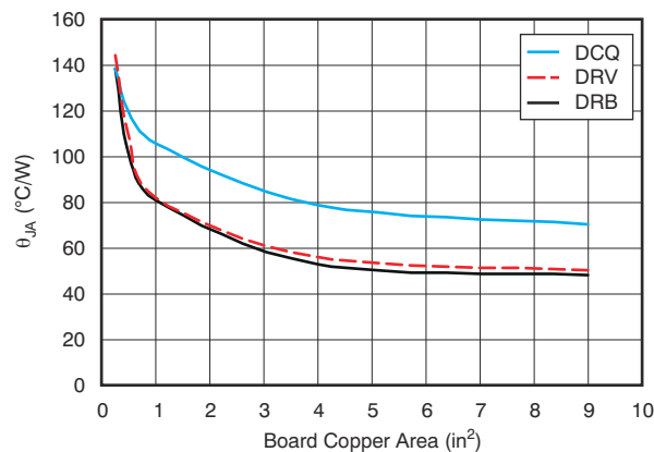
图 7-6. R_{\theta JA} vs Board Size
